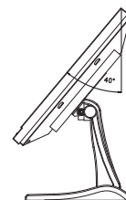
MTS17 Inclinación 40°
